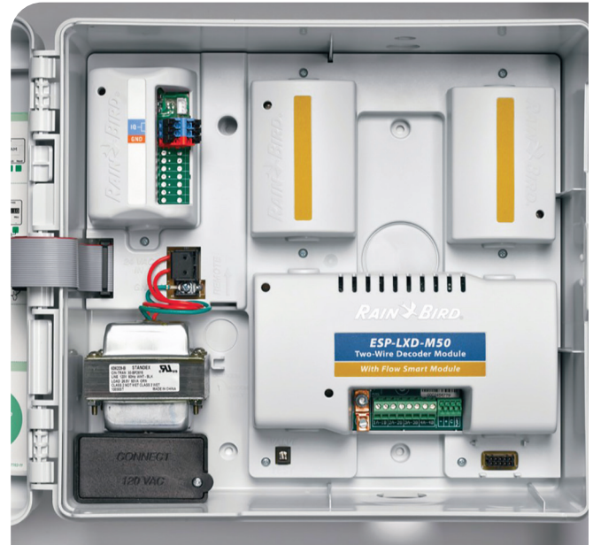
Interior del ESP-LXD con módulos
