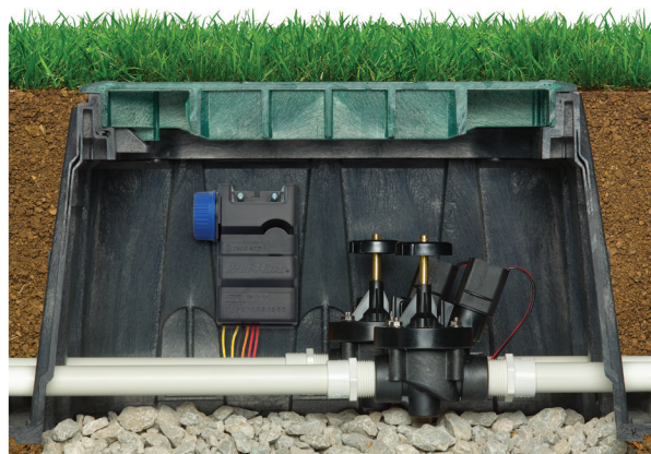
Controlador a pilas con Bluetooth y aplicación móvil TBOS-BTLT
