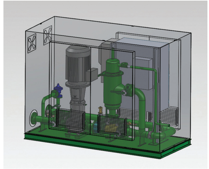
Vertical Multietapa – 1 bomba mejorada – Se muestra la caja de aluminio 5 a 50 hp; hasta 150 psi (10.3 bar); hasta 500 gpm (31.5 l/s, 114 m 3 /h)
