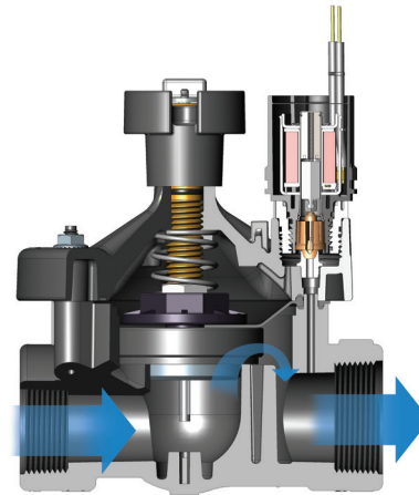
Vista transversal del modelo PEB
