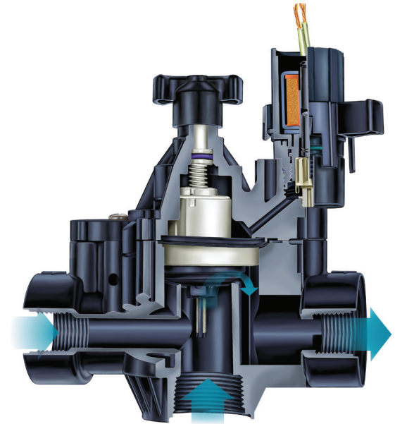
Vista transversal del modelo PGA
