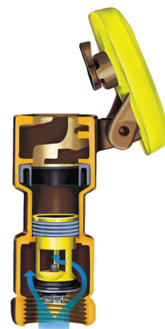
Vista transversal de una válvula de acople rápido
