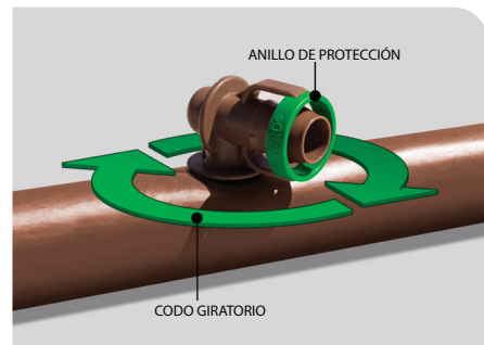
Cabezal de línea de goteo QF
