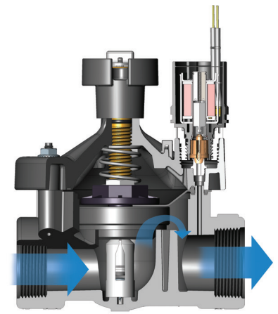
Vista transversal del modelo PESB
