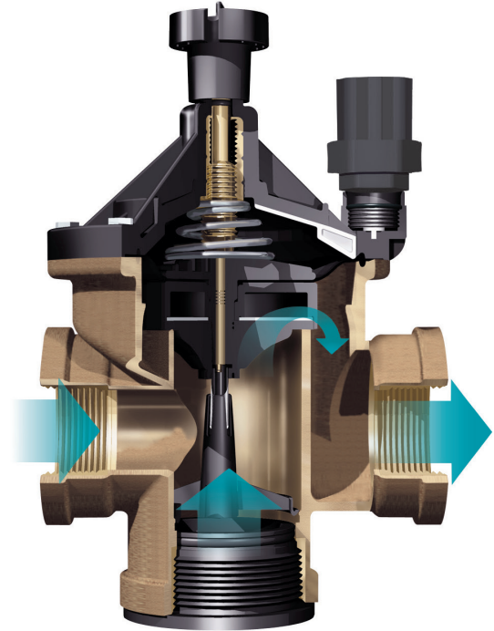
Vista transversal del modelo BPES
