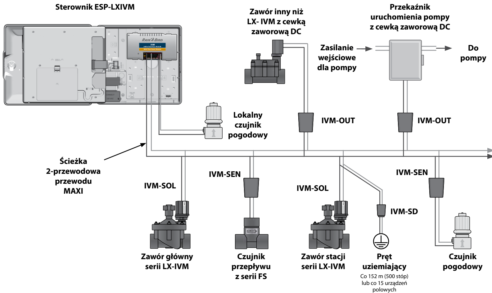
2-przewodowy system sterowania ESP-LXIVM przedstawiający połączone urządzenia IVM
